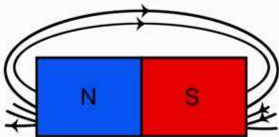
Рис. 3. Линии магнитного поля постоянного полосового магнита
