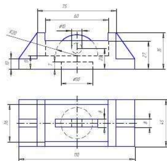
Вариант 8 Корпус
