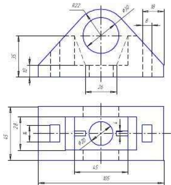
Корпус Вариант 6
