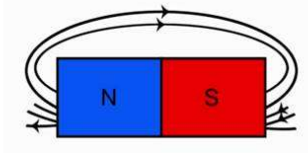
Рис. 3. Линии магнитного поля постоянного полосового магнита
