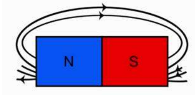
Рис. 3. Линии магнитного поля постоянного полосового магнита
